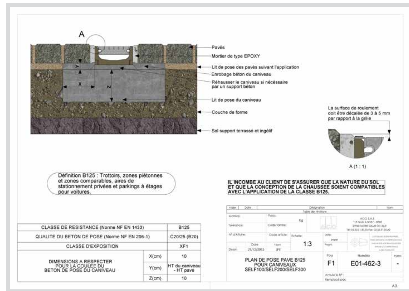
Figure 3 Plan de pose pour les caniveaux ACO Self 100, 200 et 300 avec une grille Passerelle en fonte, une grille Caillebotis ou une grille Voronoï (tous modèles), avec des pavés, classe B125
