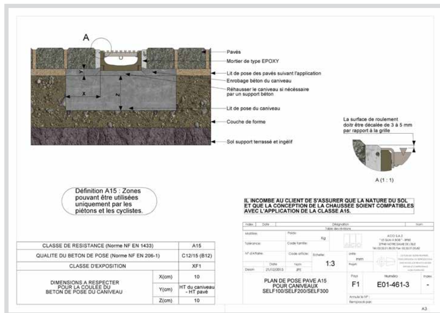
Figure 1 Plan de pose pour les caniveaux ACO Self 100 et 200 avec une grille Passerelle en acier ou polypropylène (tous modèles) ou une grille Fil inox (tous modèles) ou grille Bois (tous modèles), avec des pavés, classe A15
