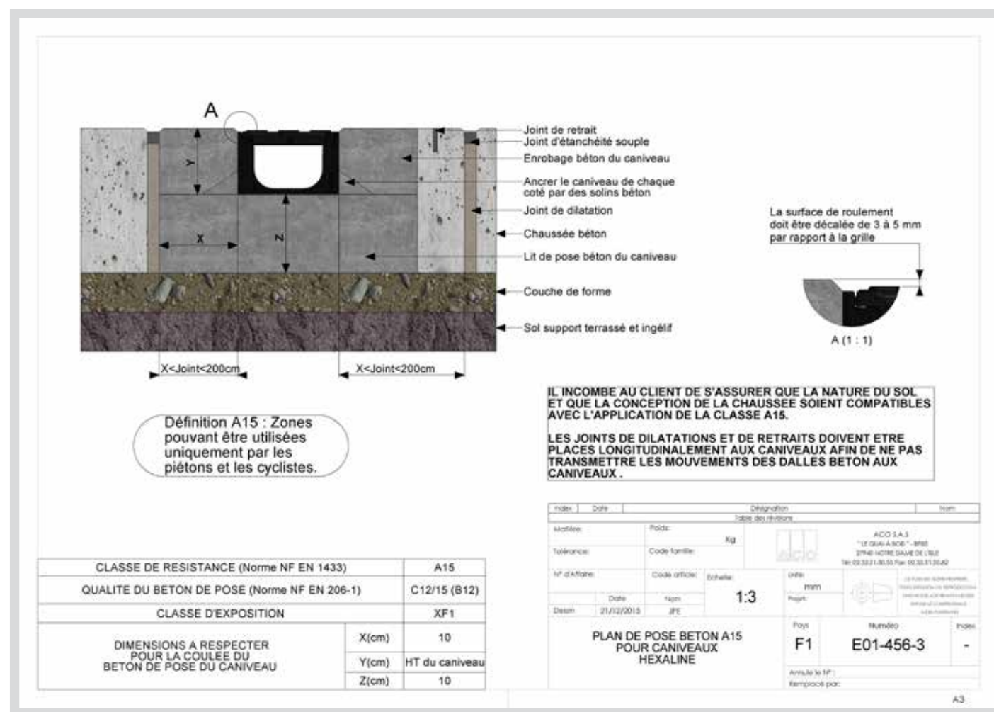
Figure 11 Plan de pose pour les caniveaux ACO Hexaline avec une grille Passerelle en acier ou polypropylène (tous modèles) ou une grille Fil inox (tous modèles), avec une dalle en béton, classe A15
