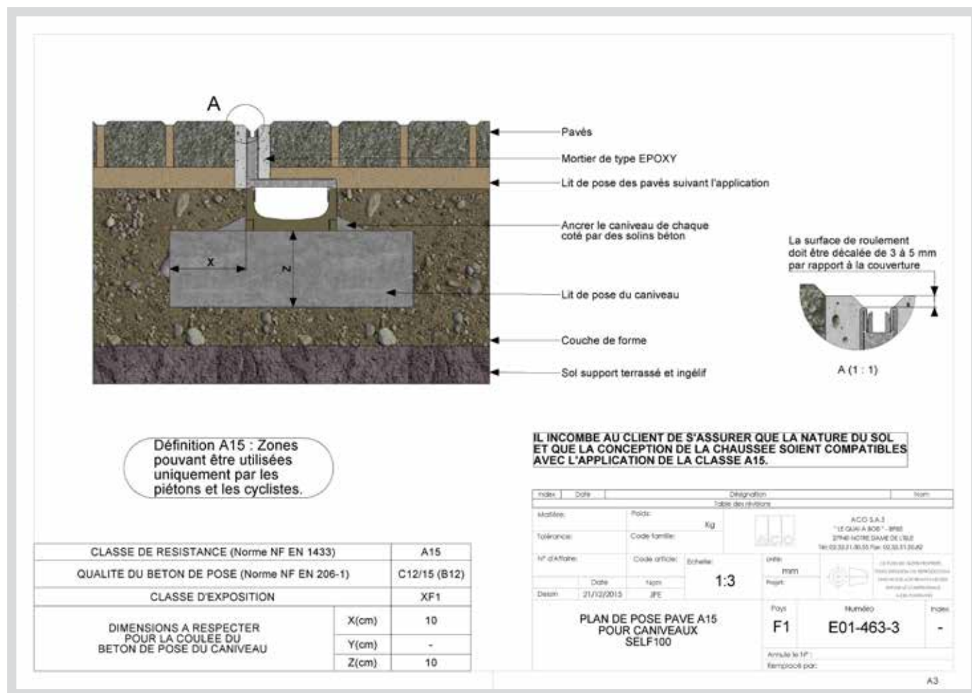
Figure 2 Plan de pose pour les caniveaux ACO Self 100 avec une couverture à fente (tous modèles), avec des pavés, classe A15
