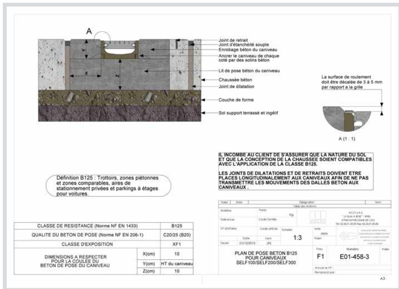
Figure 6 Plan de pose pour les caniveaux ACO Self 100, 200 et 300 avec une grille Passerelle en fonte, une grille Caillebotis ou une grille Voronoï (tous modèles), avec une dalle en béton, classe B125
