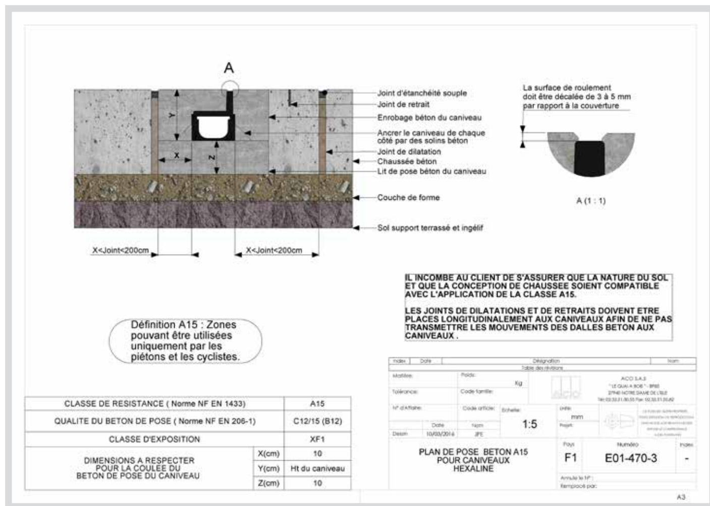
Figure 12 Plan de pose pour les caniveaux ACO Hexaline avec une couverture à fente (tous modèles), avec une dalle en béton, classe A15
