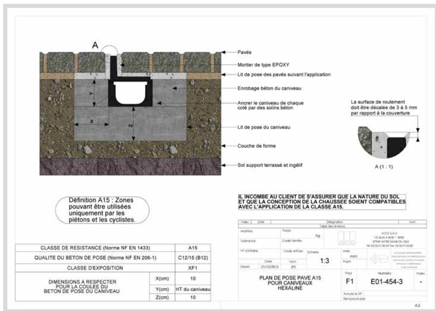
Figure 10 Plan de pose pour les caniveaux ACO Hexaline avec une couverture à fente (tous modèles), avec des pavés, classe A15
