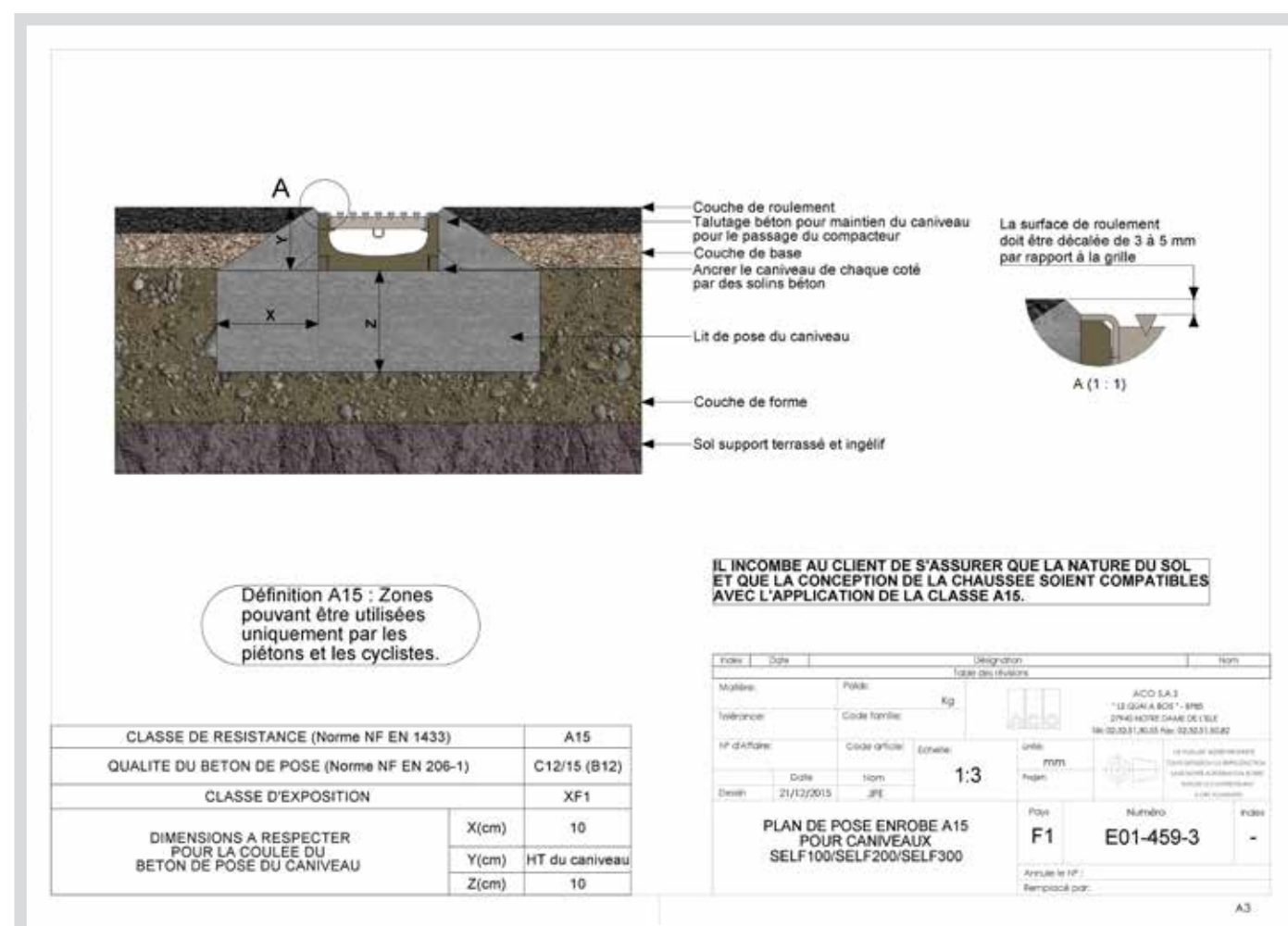
Figure 7 Plan de pose pour les caniveaux ACO Self 100 et 200 avec une grille Passerelle en acier (tous modèles), une grille Fil inox (tous modèles) ou une grille Bois (tous modèles), avec un enrobé ou un asphalte, classe A15
